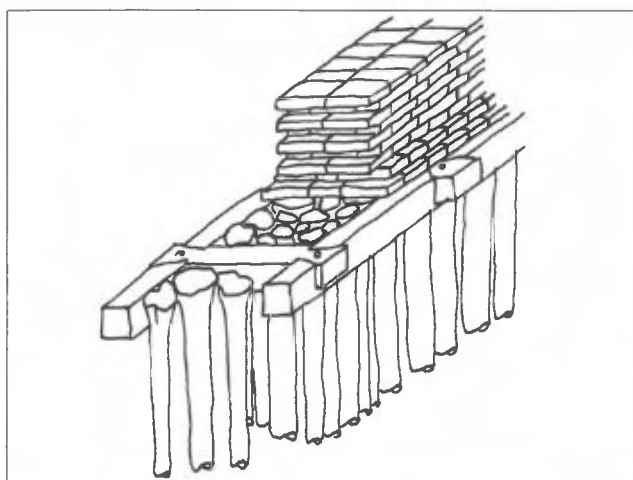
Afb. 16. Funderingsprincipe tweede stadsmuur (S87) (naar Gawronski en Veerkamp 2003, 18 Tek: R. Tousain BMA).
